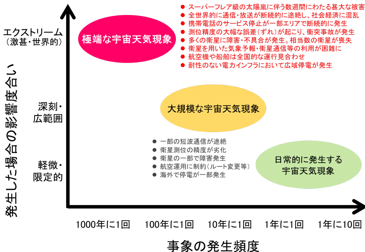
図 11 宇宙天気リスクのランドスケープ（俯瞰図）
