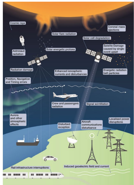
図5 宇宙天気がもたらす影響（同対処戦略より）
