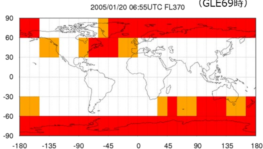
ICAOアドバイザリ作成に利用される被ばく線量マップ (GLE69時)
